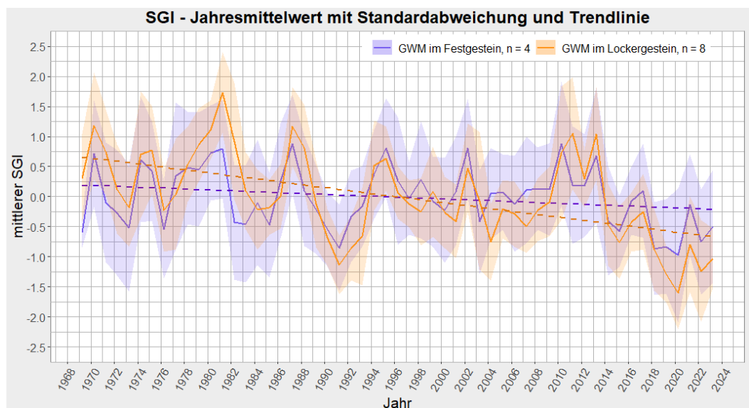
Abbildung 2: Mittlerer jährlicher Standard-Grundwasser-Index (SGI), sowie dessen Standardabweichung und linearer Trend im Fest- und Lockergestein von Sachsen im Zeitraum 11/1970 – 03/2023 (Festgestein 4 GW-Messstellen, Lockergestein 8 GW-Messstellen)
